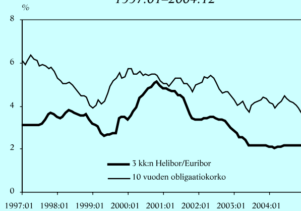
Korot 1997:01–2004:12
